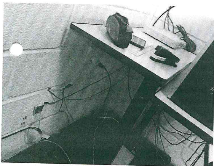
Figura 3: Fiação exposta e com conexões perigosas.
